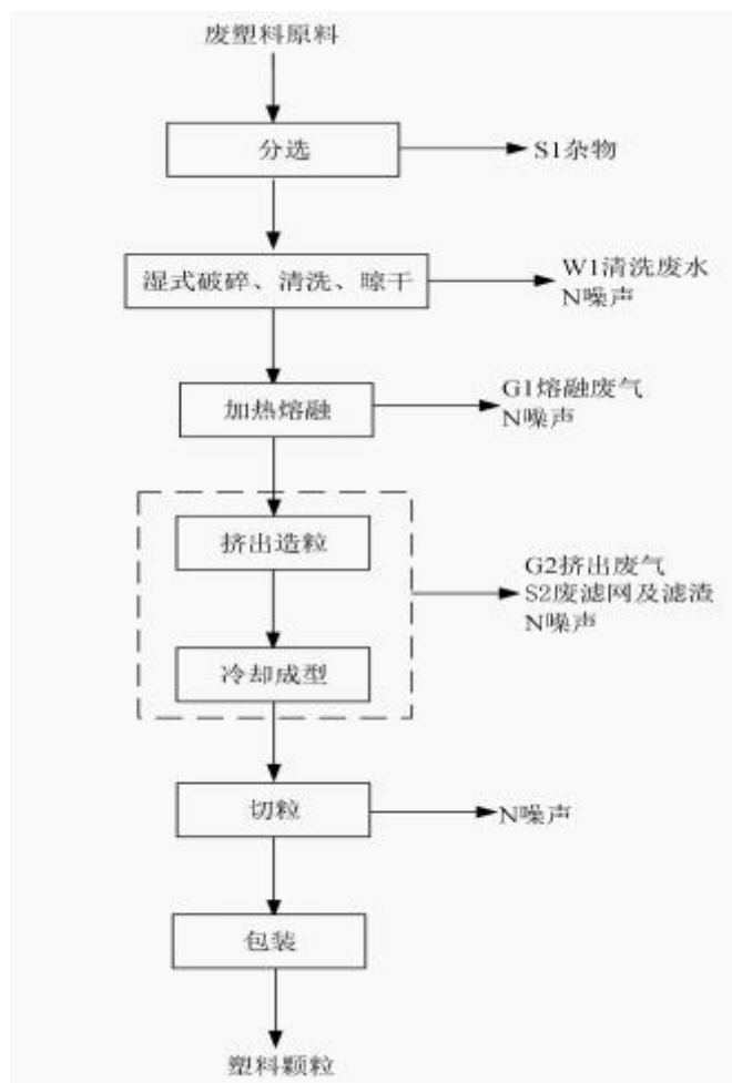
图 3-2 造粒生产工艺流程图
