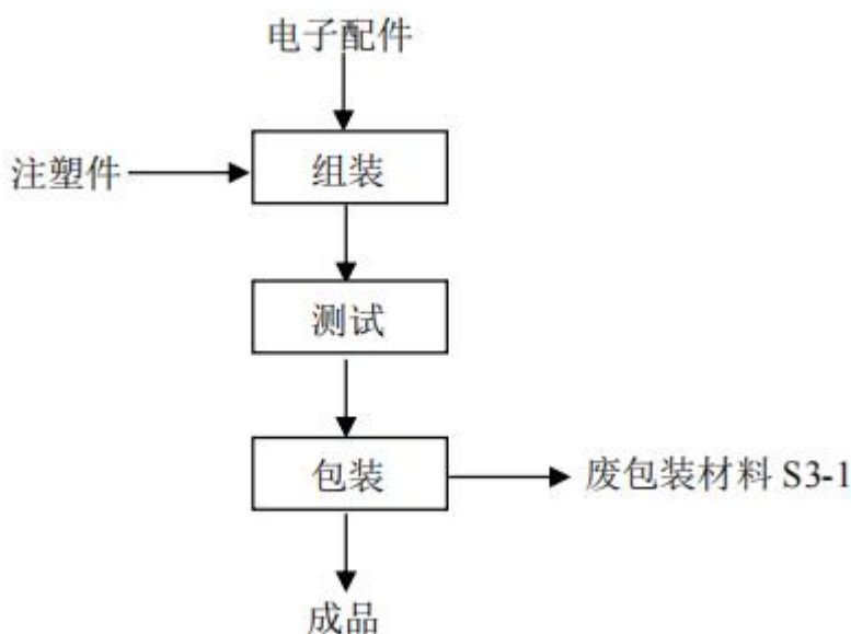
图 3-3 光通讯产品结构件、电子零部件生产工艺流程及产污环节图
